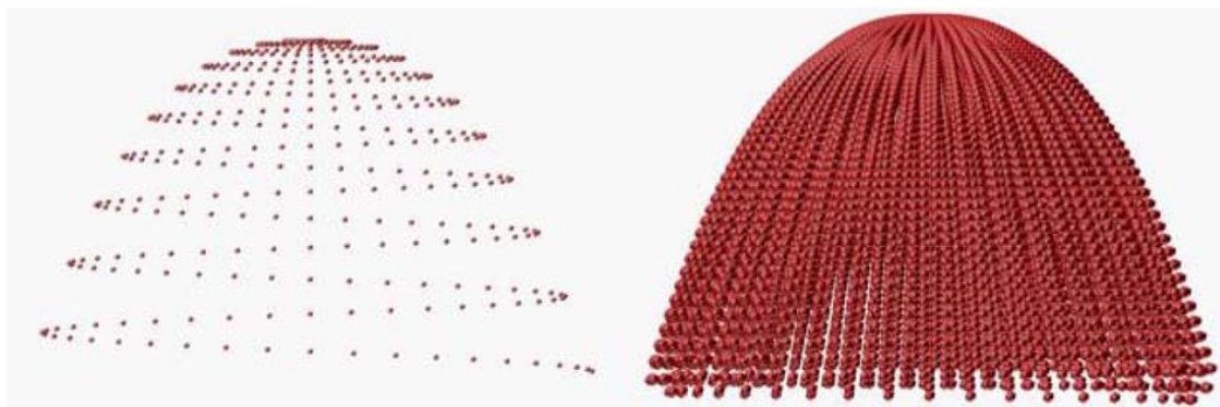
Фиг. 2.5 Лёгкие атомные и «тяжёлые» СВЧ – фотоны.
