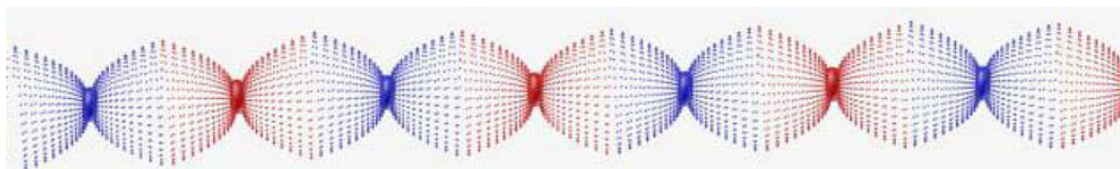
Фиг. 2.3 Трек фотона
