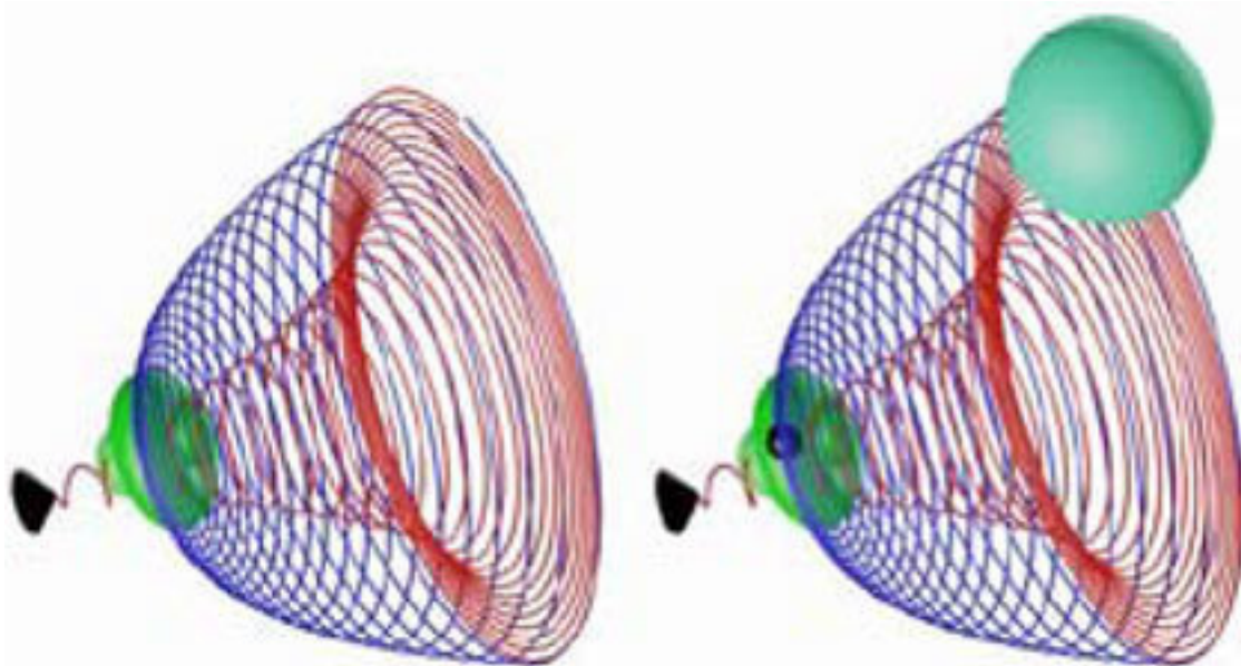
Фиг. 2.9 Схема процесса регенерации магнитного монополя гравитационным.
