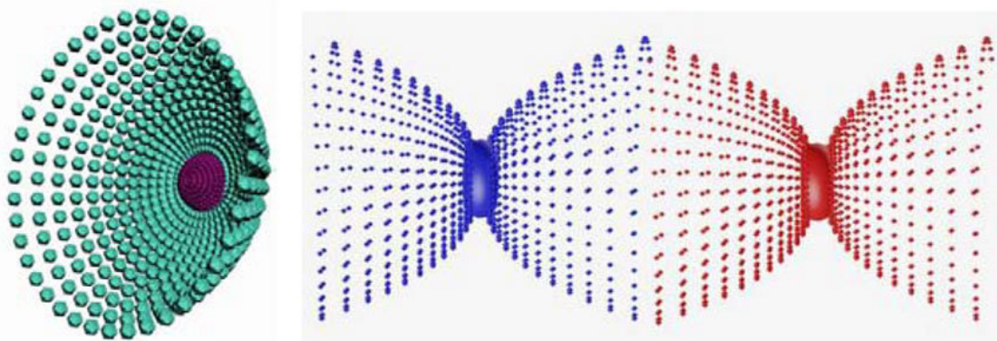
Фиг. 2.2 Схема волновода фотона из зёрен-электропотенциалов.
