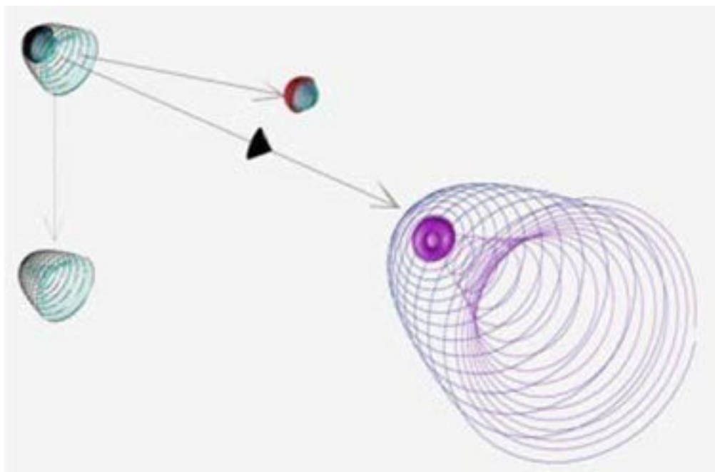
Фиг. 2.10 Распад нейтрона
