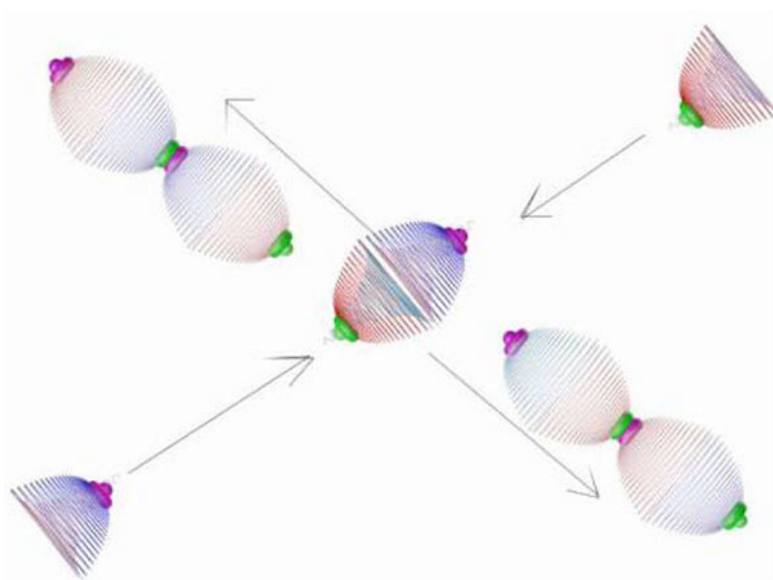
Фиг.2.12 Схема аннигиляция электрона и позитрона
