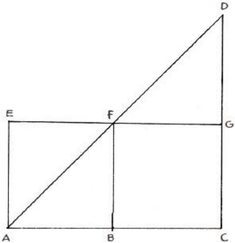
Рис. 7. Найденное Оремом графическое доказательство теоремы о средней скорости. Горизонтальная ось AC озна-
