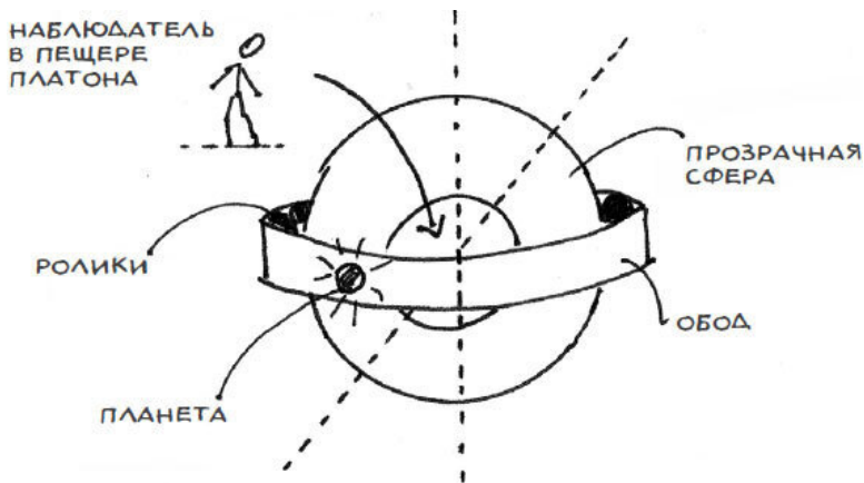
Рис. 5. Движение планет в модели Евдокса
