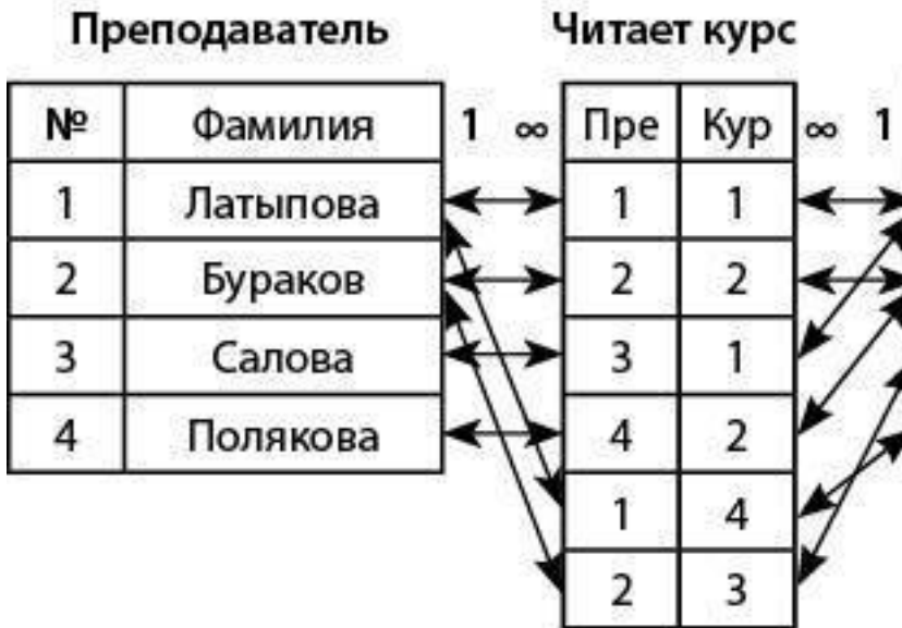
Рис. 9. Преобразование связи «многие-ко-многим»
