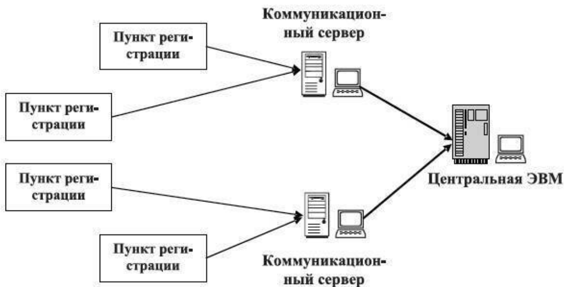
Рис. 3.6. Метод сбора первичной информации в регламентном режиме
