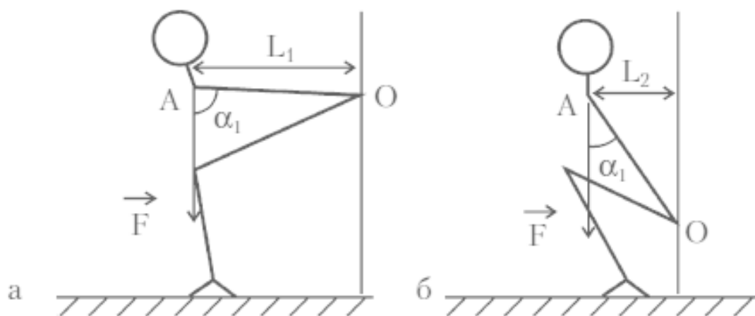
Рис. 16. Нагрузка, которая приходится на спину при различных стартовых положениях: а – старт «спиной»; б – старт «ногами»
