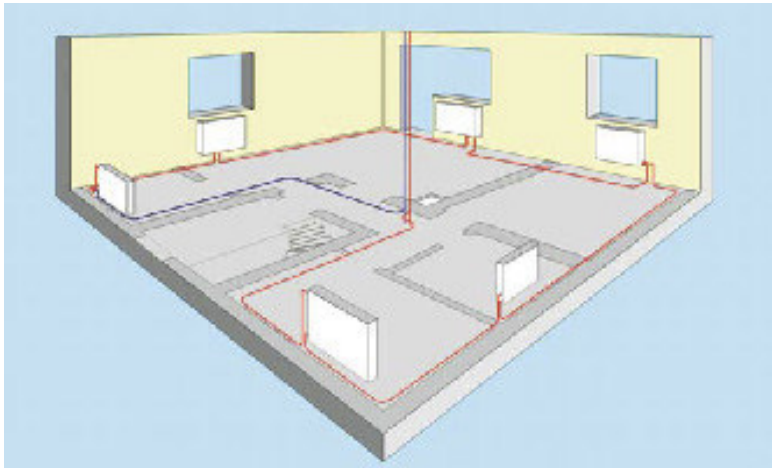
Рис. 1. Пример однотрубной разводки
