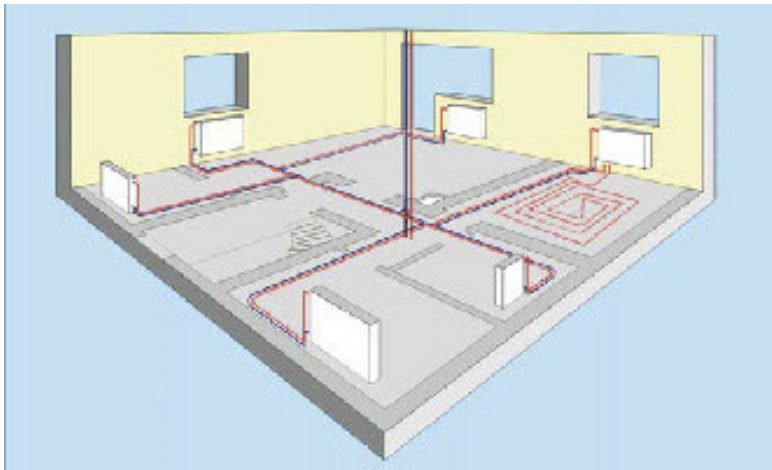
Рис. 2. Двухтрубная схема с центральной распределительной магистралью
