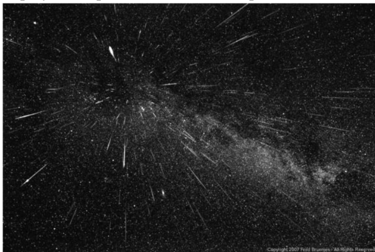
Рис. 2.1. Метеорный поток Персеиды ( http://www/moonglow.net/ccd/pictures/meteors/index.html )
