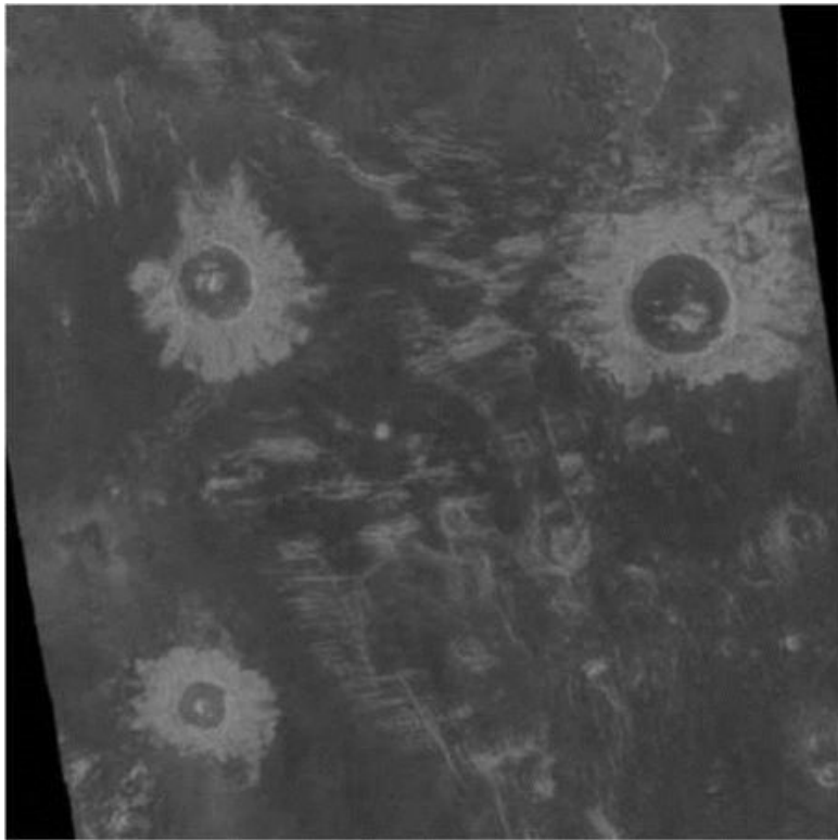
Рис. 2.12. Поверхность Венеры ( http://pds.jpl.nasa.gov/planets/captions/venus/ )
