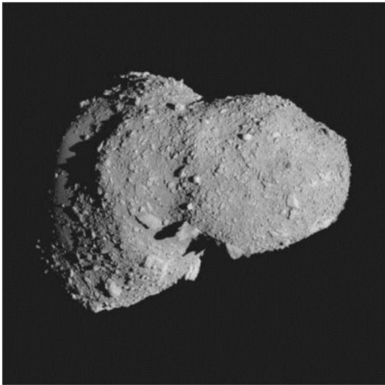
Рис. 2.16. Астероид Итокава ( http://galspace.spb.ru/ )
