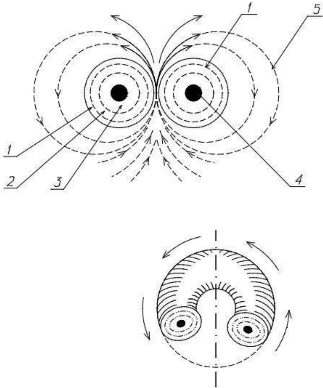
Рис.2. Структура Черной дыры. 1, 2, 3 – слои с последовательным повышением частоты ЕЭМ – кипящие потоки рождения и аннигиляции нейтринных пар. 4 – сердцевина Черной дыры. 5- магнитное поле Черной дыры.
