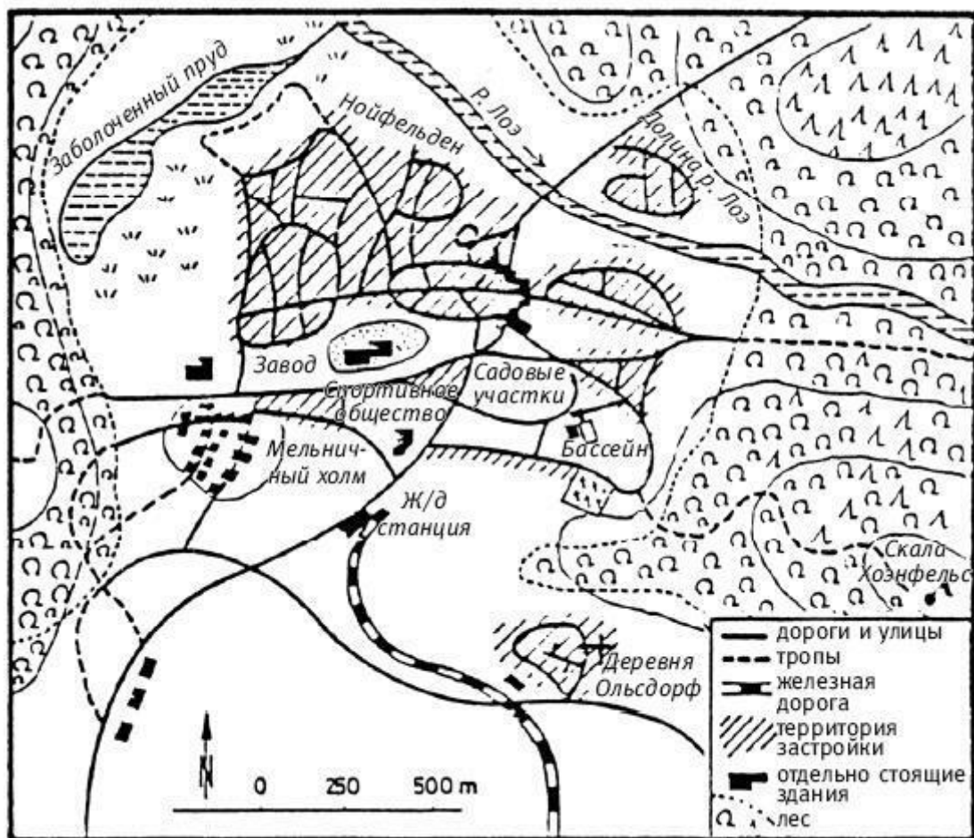
Рис. 8. План города Лоххаузена
