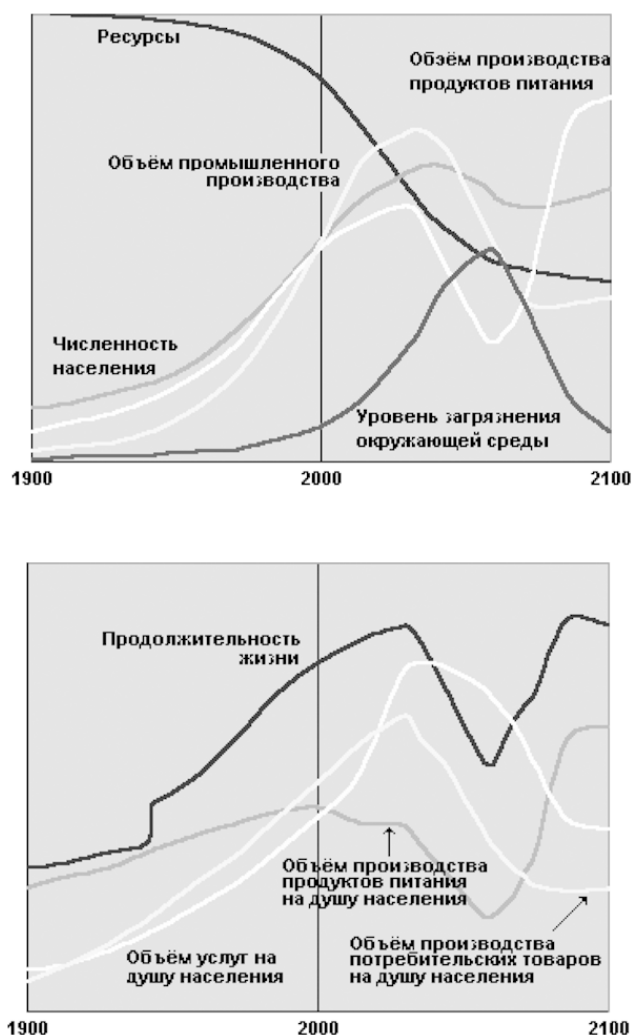
Рис. 3. Сценарий 12 из книги «За пределами роста».
