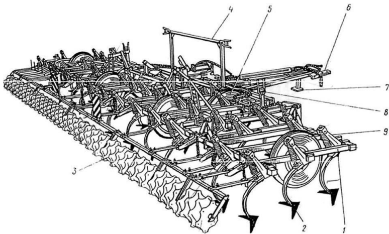
Рисунок 3.2 – Культиватор КШУ-12 (в рабочем положении):
