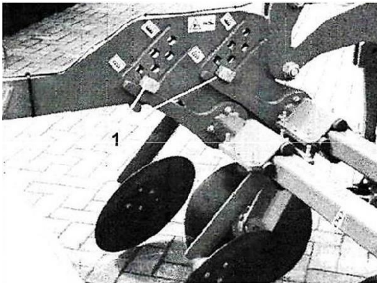
Рисунок 2.6 – Регулятор глубины сферических дисков: 1 – эксцентриковый палец
