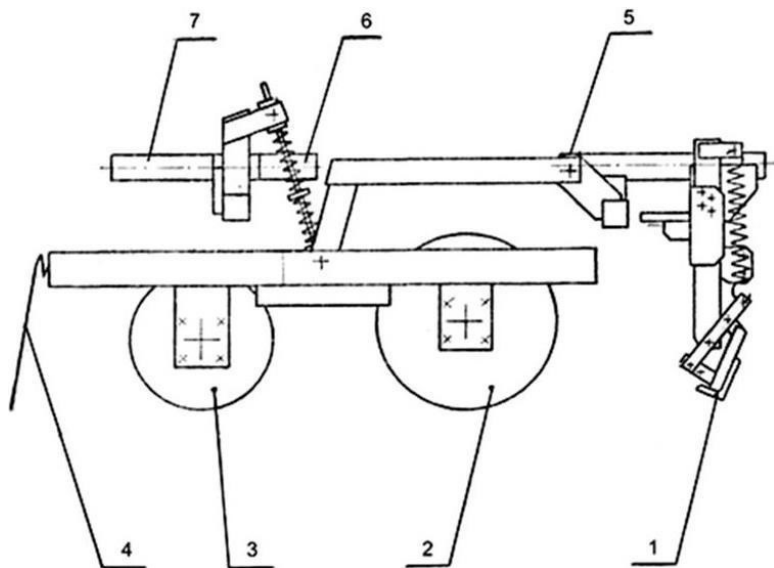
Рисунок 1.4 – Прикатчик: 1 – волокуша; 2 – каток угловый; 3 – каток угловый; 4 – зубья пружинные; 5, 6, 7 – втулки
