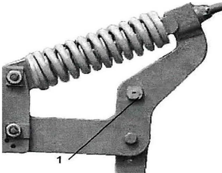
Рисунок 2.8 – Лапа с пружинным предохранителем:
