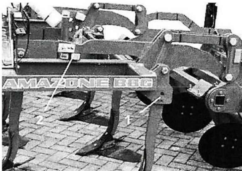
Рисунок 2.5 – Срезной болт: 1 – срезной болт; 2 – четырёхгранный эксцентриковый палец
