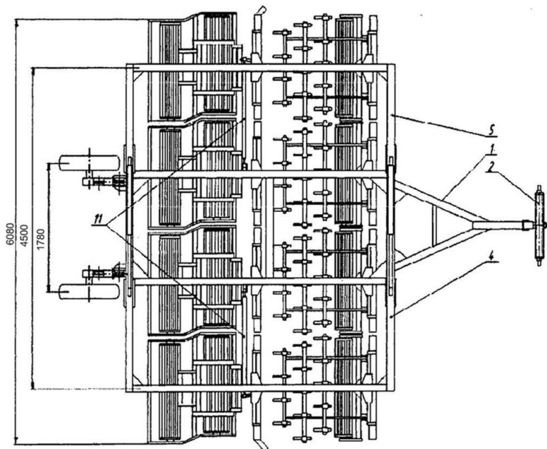
Рисунок 1.1 – Культиватор комбинированный КППШ-6: 1 – рама средняя; 2 – траверса; 3 – шасси; 4 – рама правая; 5 – рама левая; 6 – секция культиваторная; 7 – прикатчик; 8 – следорыхлитель; 9 – цепь; 10 – стойка опорная; 11 – тя-
