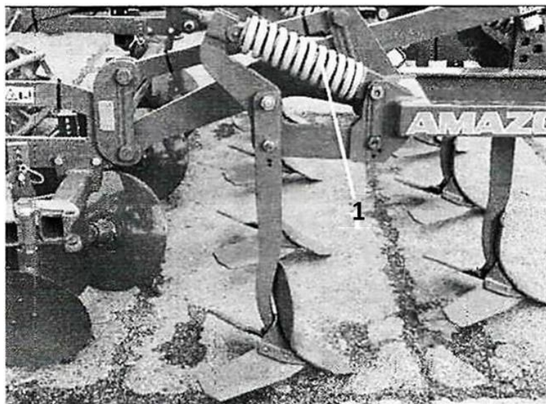
Рисунок 2.3 – Пружинный предохранитель: 1 – пружина
