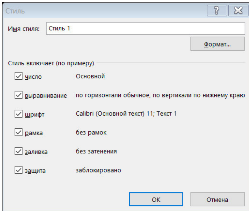
Рисунок 3. Окно «Стиль»
