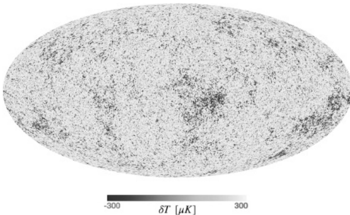
Рис. 2. Послесвечение горячего Большого взрыва. Это тепловая карта неба на микроволновых частотах, построенная по данным названного в честь основателя квантовой физики Макса Планка спутника «Планк» Европейского космического агентства. Сгущения различных оттенков серого соответствуют малым изменениям температуры реликтового космического микроволнового излучения, приходящего к нам с разных направлений на небе. На первый взгляд распределение этих температурных флуктуаций выглядит случайным, но тщательный анализ выявил в нем структуры, связывающие друг с другом различные участки карты. Исследуя эти структуры, космологи могут реконструировать историю расширения Вселенной, построить модель образования в ней галактик и даже предсказать ее будущее.
