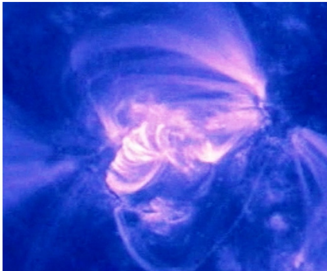
Фото 9. Магнитный диполь в хромосфере Солнца
