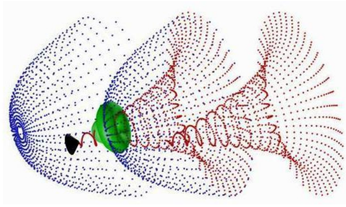
Фото 11. Пульсации обновлённых магнитным монополем контуров электрона при формировании его внешнего поля
