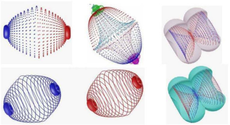
Фото 17. Схемы \pi – мезонов и структуры их волноводов.
