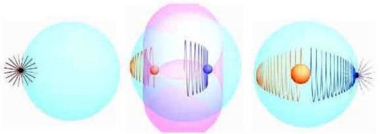
Фото 8. Изменения магнитного поля в фазовом объёме полволны
