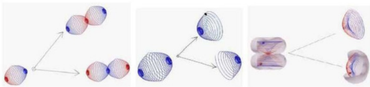
Фото 18. Распады мезонов, слева нейтрального, справа заряженных.
