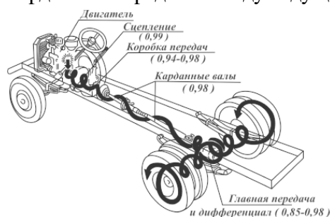
Рис. 2. Схема усилия от двигателя к колесам автомобиля. Цифры в скобках означают коэффициенты полезного действия отдельных механизмов
