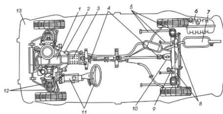
Рис. 1. Общая компоновка заднеприводного автомобиля ВАЗ 2105 с расположением двигателя спереди: 1 – двигатель; 2 – сцепление; 3 – коробка передач; 4 – карданная передача; 5 – детали задней подвески; 6 – топливный бак; 7 – глушитель; 8 – амортизаторы; 9 – задний мост; 10 – главная передача и дифференциал; 11 – рулевое управление; 12 – детали передней подвески; 13 – кузов
