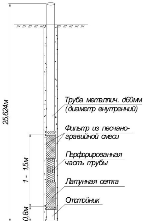
Рис. 1. Конструкция скважины
