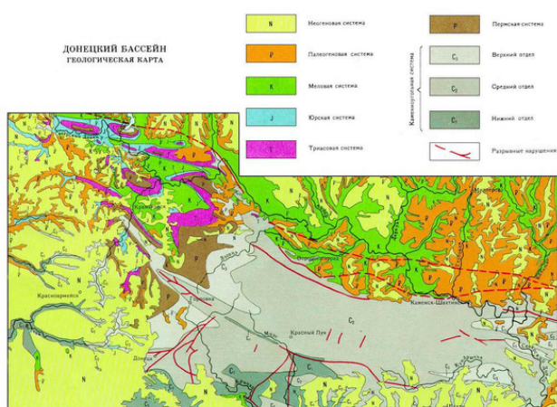
Геологическая карта Донецкого каменноугольного бассейна
